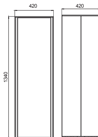
Pohľad spredu
