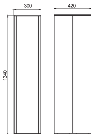
Pohľad spredu
