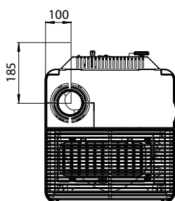
Pohľad zhora
