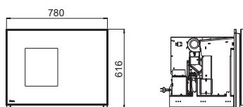
E15554 okolitý kryt úzky čierny
